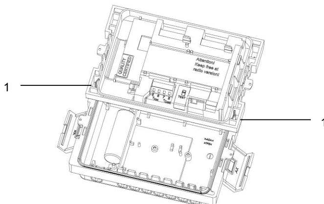
Bild DD Installationsläge för överdel
