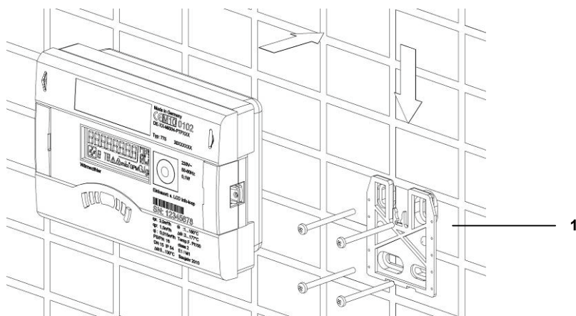
Bild W Vägghäring
