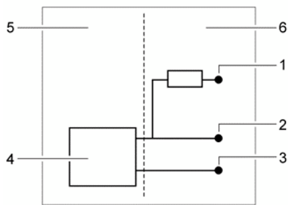
Bild M Kopplingsschema för pulsutgång
