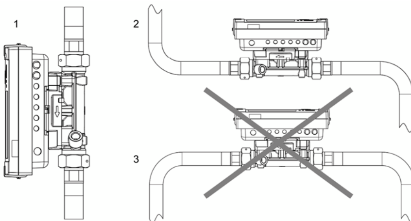
Bild S Installationslägen
