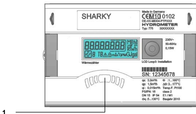
Bild D Framsidan på räknaren
